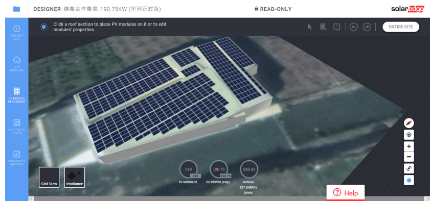
SolarEdge Designer 中的傑農農場屋頂型系統的 3D 設計
