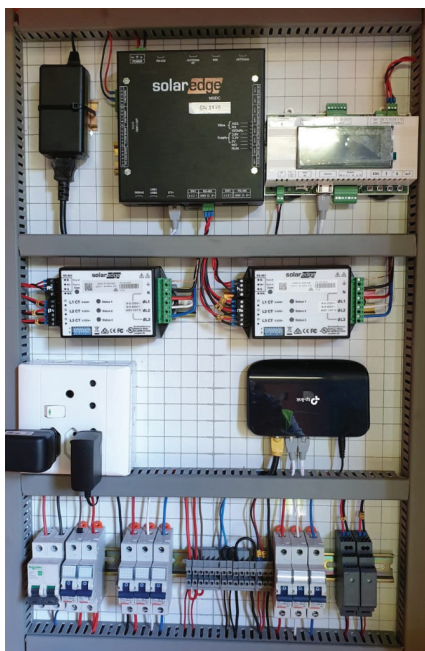
ディーゼル発電機(550kVa)を使用した341kWp 太陽光発電設置(南アフリカ)
