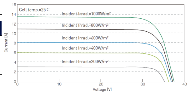
Module I-V Curve
