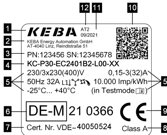
Fig. 4-7: Typeskilt (eksempel)
