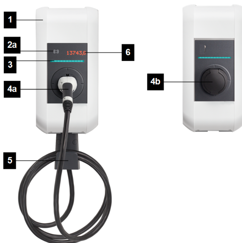
Fig. 4-4: Oversikt ladestasjon
