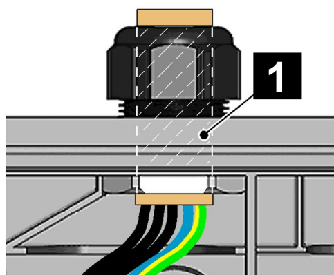
Korrekt kabelgjennomføring (åpen kabelmontering)
