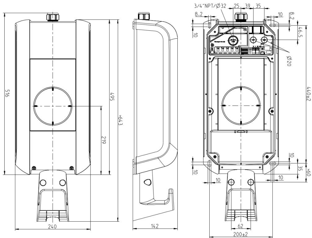
Fig. 13-21: Mål i mm
