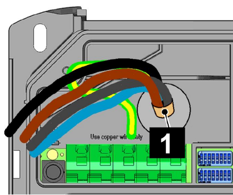
Dobbeltmembranstusser (skjult kabelmontering)
