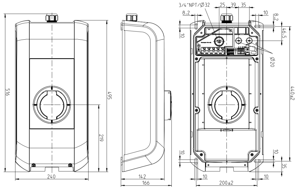
Fig. 13-20: Mål i mm
